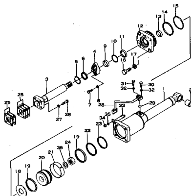
Fig. 111 テルトシリンダ (通称号機) TILT CYLINDER (Serial No. 2001~)
