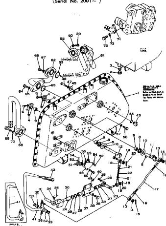
Fig. 131 ハイドロリック タンク 取付 コントロール レバー HYDRAULIC TANK AND CONTROL LEVER (Serial No. 2001-)
