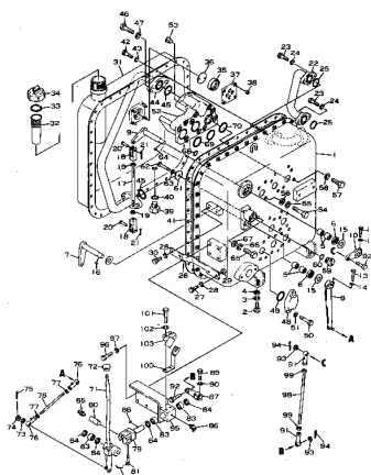
ハイドロリック タンク および コントロール レバー Fig. 103 HYDRAULIC TANK AND CONTROL LEVER DDC050-1A1C / 適用 号 機 DDR050-1A1B (Serial No. 1001 ~ )
