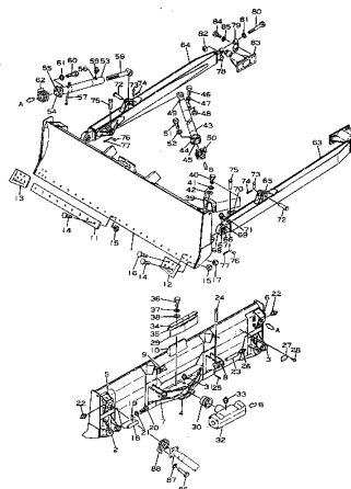
Fig. 107 TILT BLAD DDR050-1A (Serial No. 1001 ~ 1053)
