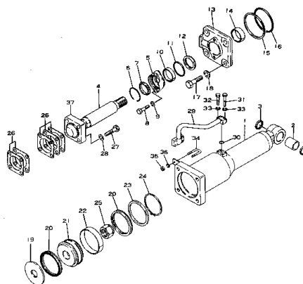
チルト シリンダ Fig. 102 TILT CYLINDER DDC050-1A,1C (適用号機 DDR050-1A,1B (Serial No. 1001~))
