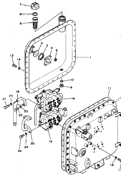
ハイドロリック タンク Fig. 131 HYDRAULIC TANK (1/2)
