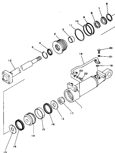
Fig. 111 テルトシリンダ TILT CYLINDER
