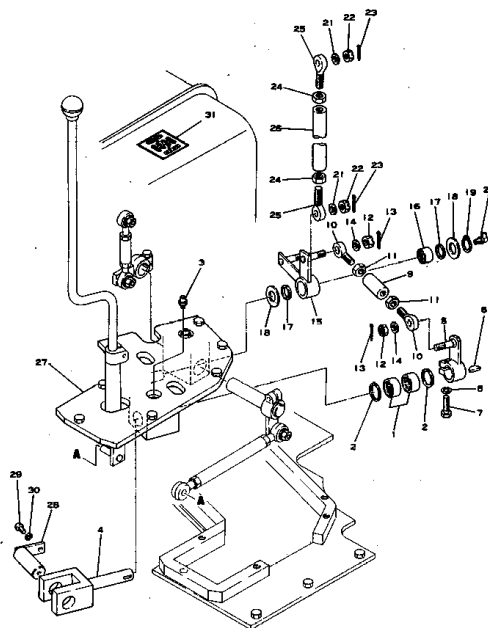
ブレード および トリミング コントロール レバー Fig. 103 BLADE AND TRIMMING CONTROL LEVER
