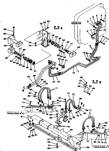
トリミング パイピング Fig. 104 TRIMMING PIPING
