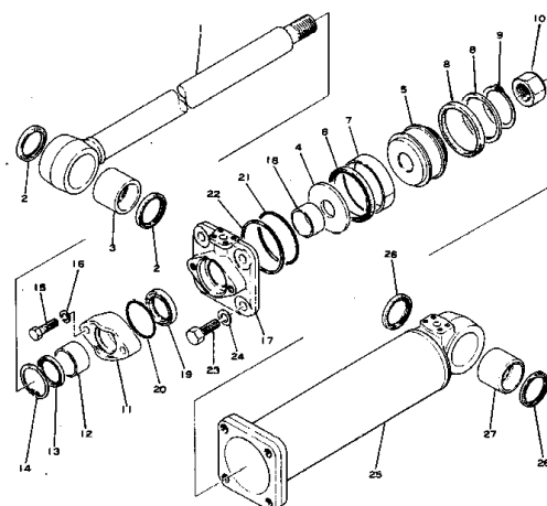
トリミング シリンダ Fig. 106 TRIMMING CYLINDER
