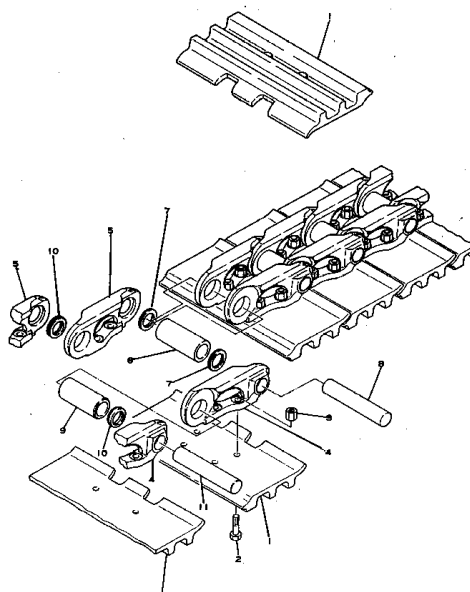
Fig. 108 トラック シュー (トリプル グローサ) TRACK SHOE (TRIPLE GROUSER)
