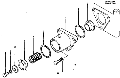
リターン スプリング ケース Fig. 102 RETURN SPRING CASE
