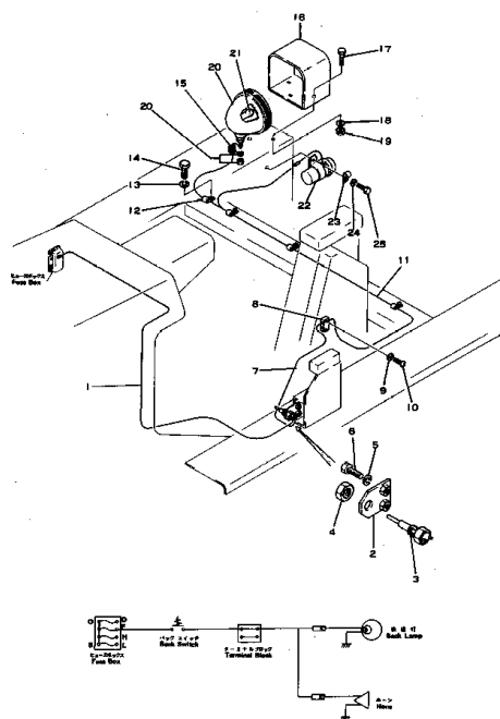
Fig. 107 バック ホーン および バック ブザー BACK HORN AND BACK BUZZER
