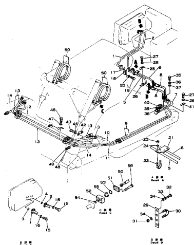
Fig. 221 ハイドロリック オイル パイピング Fig. 221 HYDRAULIC OIL PIPING
