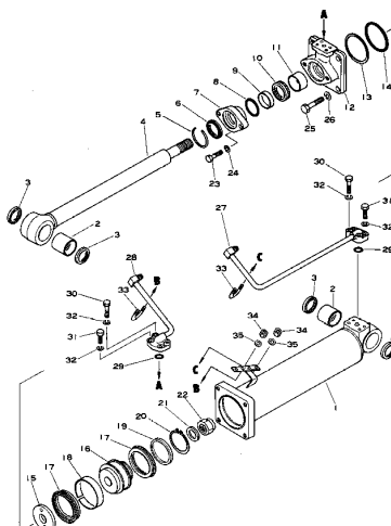
ブレードトリミングシリンダ Fig. 111 BLADE TRIMMING CYLINDER
