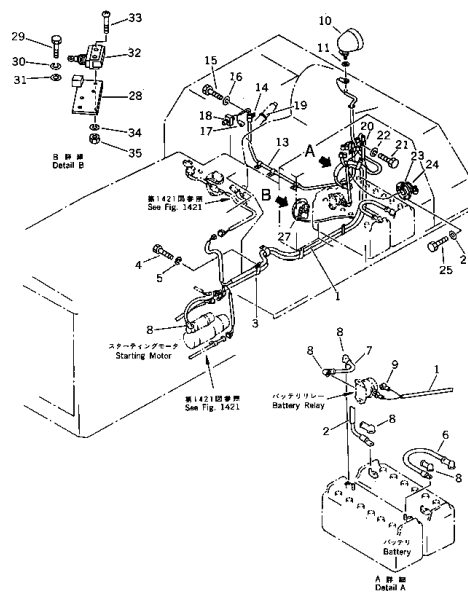
エレクトリカル システム トリミングドーザー用 FIG. 1427 ELECTRICAL SYSTEM (2/2) (FOR TRIMMING DOZER) 適用号機 (D41A SERIAL NO. 10001-)
