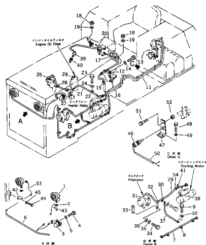
エレクトリカル システム トリミングドーザー用 FIG. 1426 ELECTRICAL SYSTEM (1/2) (FOR TRIMMING DOZER) 適用機 (D41A SERIAL NO. 10001-)
