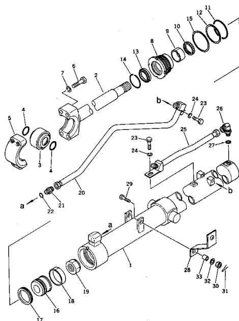
ブレード リフト シリンダ Fig. 113 BLADE LIFT CYLINDER
