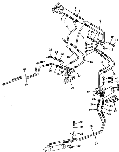
ハイドラリック パイピング Fig. 121 HYDRAULIC PIPING
