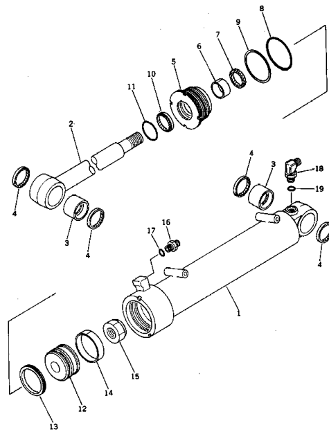
ブレード トリミング シリンダ Fig. 111 BLADE TRIMMING CYLINDER
