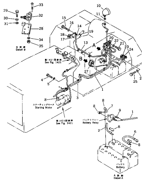
エレクトリカル システム トリミングドーザー用 FIG. 1427 ELECTRICAL SYSTEM (2/2) (FOR TRIMMING DOZER) 適用機種 (D41A SERIAL NO. 10001-)
