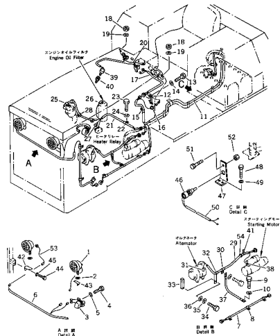
エレクトリカル システム トリミングドーザー用 FIG. 1426 ELECTRICAL SYSTEM (1/2) (FOR TRIMMING DOZER) 適用機 (D41A SERIAL NO. 10001-)
