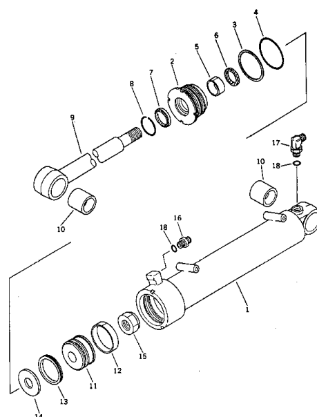
ブレードトリミングシリンダ Fig. 211 BLADE TRIMMING CYLINDER
