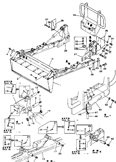
トリミング ブレード Fig. 111 TRIMMING BLADE (DDM030-2B,2C)
