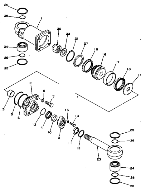
FIG. 112 ブレードチルトシリンダ BLADE TILT CYLINDER
