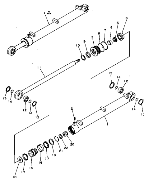
FIG. 111 ブレード アングル シリンダ BLADE ANGLE CYLINDER
