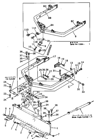
FIG. 101 BLADE FRAME
