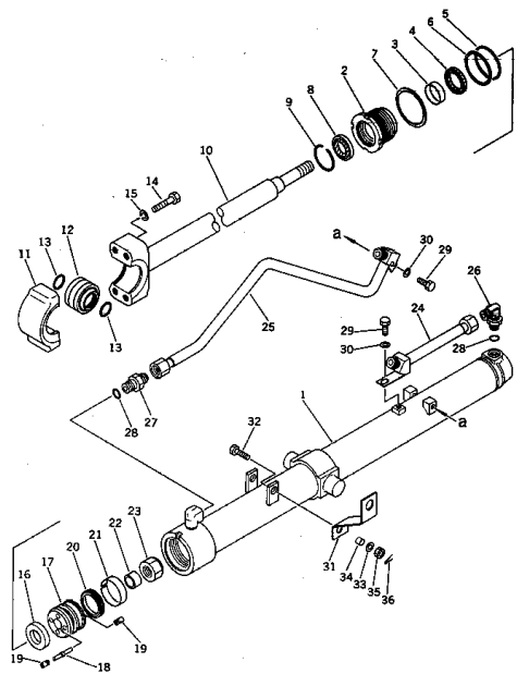
Fig. 111 ブレード リフト シリンダ BLADE LIFT CYLINDER
