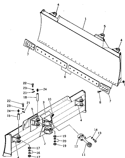
ブレード Fig. 101 BLADE
