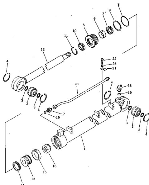
ブレード アングル シリンダ Fig. 115 BLADE ANGLE CYLINDER
