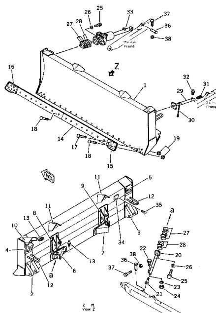
ブレード (適用機種 Fig. 101A BLADE (Serial No. (80001~))
