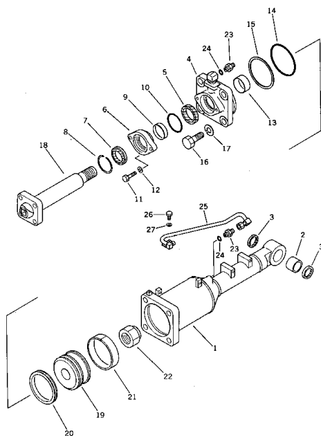
Fig. 111A テルト シリンダ (適用機種: (80001~)) TILT CYLINDER (Serial No. (80001~))
