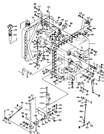
ハイドロリック タンク および コントロール レバー Fig. 103 HYDRAULIC TANK AND CONTROL LEVER DDC050-1A1C / 適用 号 機 DDC050-1A1B (Serial No. 1001 ~ )
