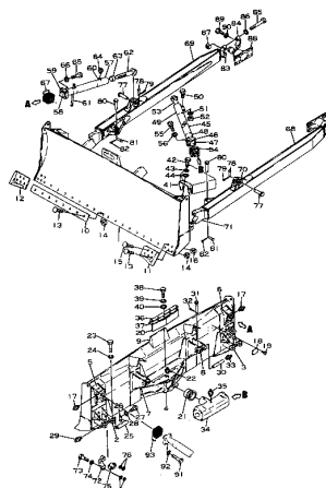
Fig. 101A TILT BLADE DDC050-1C (適用機種 Serial No. 1035 ~)
