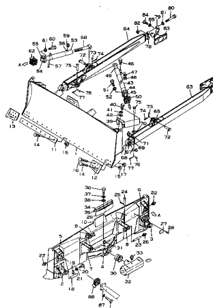
チルトブレード Fig. 101 TILT BLADE (適用機種 DDC050-1A (Serial No. 1001 ~ 1034))
