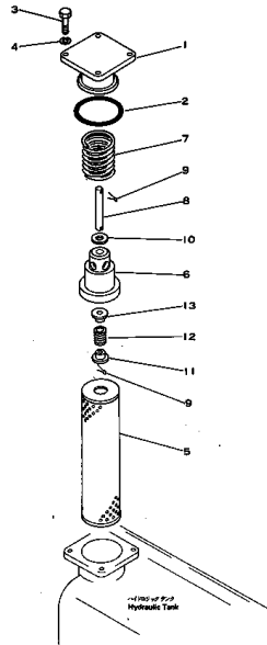
ハイドロリック フィルタ Fig. 123 HYDRAULIC FILTER
