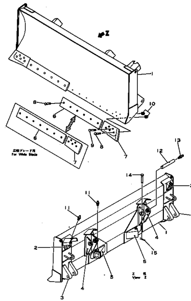
Fig. 101 ストレート チルト ブレード STRAIGHT TILT BLADE
