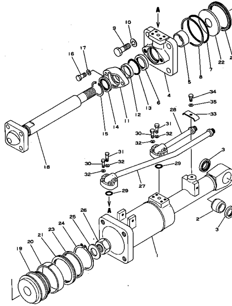
ブレード チャルト シリンダ Fig. 111 BLADE TILT CYLINDER
