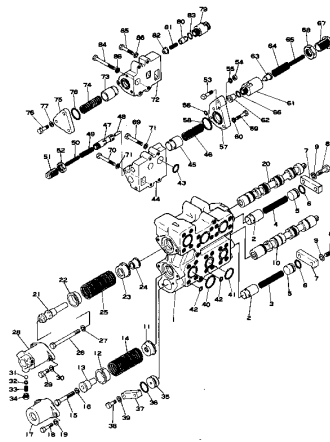
Fig. 104 バケツコントロールバルブ BUCKET CONTROL VALVE
