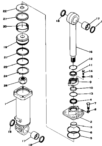
クラムシェル シリンダ Fig. r192 CLAMSHELL CYLINDER
