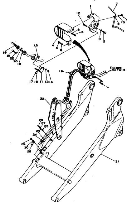
ハイドロリックパイピング 車体側 (1/2) Fig. 185 HYDRAULIC PIPING (CHASSIS SIDE) (1/2) (適用号機 (Serial No. (5022-))
