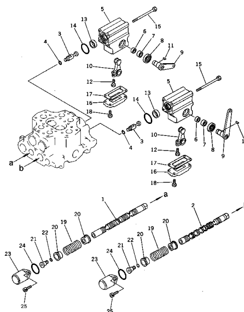
Fig. 136 ハイドロリック コントロール バルブ HYDRAULIC CONTROL VALVE (2/3)
