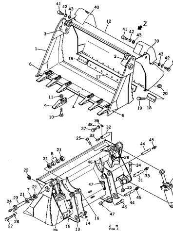
Fig. 101 バケット BUCKET
