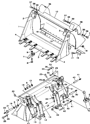
Fig. 101 バケット BUCKET
