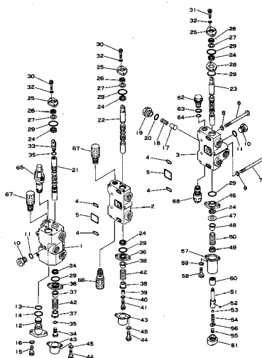
コントロールバルブ Fig. 145 CONTROL VALVE(1/3)
