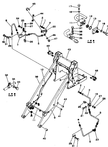
パイピング (コントロールバルブ→リフトアーム) Fig. 121 PIPING(1/2) (Control Valve→Lift Arm)
