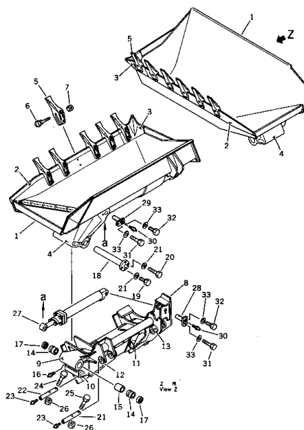
バケット および サポート Fig. 101 BUCKET AND SUPPORT (DBD053-1A)
