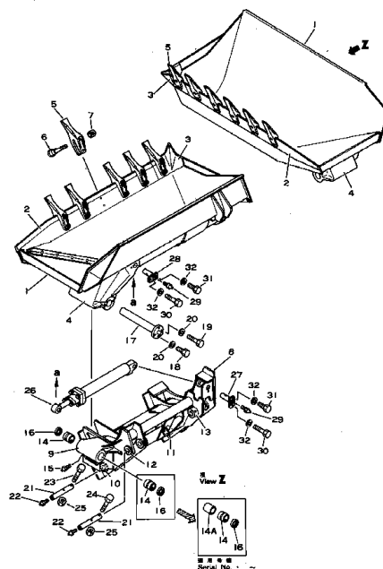
Fig. 101 バケツ および サポート (DBD050-2C, DBD057-1A)
