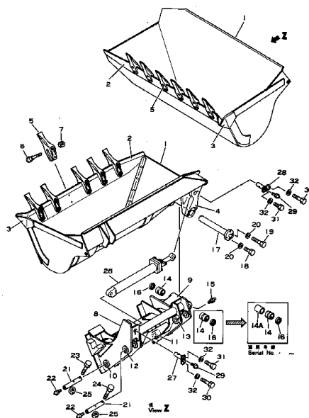
バケット および サポート Fig. 102 BUCKET AND SUPPORT (DBD050-2D, DBD057-1B)
