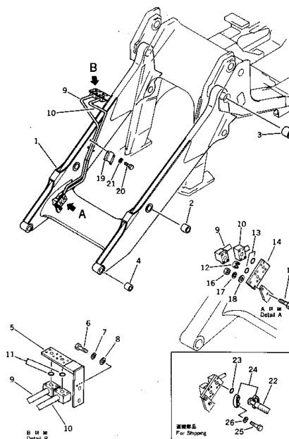
ハイドロリックパイピング Fig. 122 HYDRAULIC PIPING (2/3)
