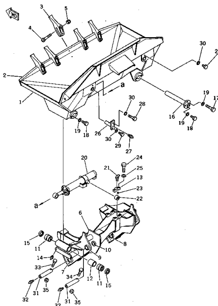
バケット および サポート Fig. 101 BUCKET AND SUPPORT
