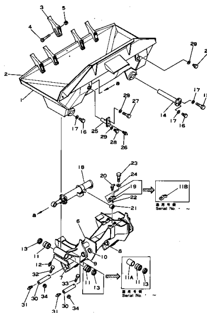
バケット および サポート Fig. 101 BUCKET AND SUPPORT
