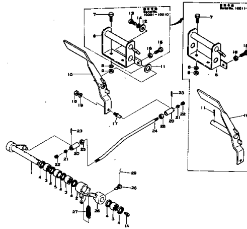
Fig.1111 DECELERATOR PEDAL (トルクフロー式、適用号機 )
