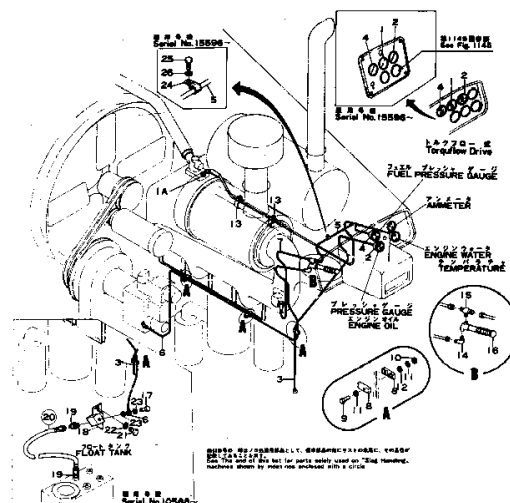
エンジン関連部品 Fig.1101 ENGINE RELATED PARTS (適用機種 10001~ )
