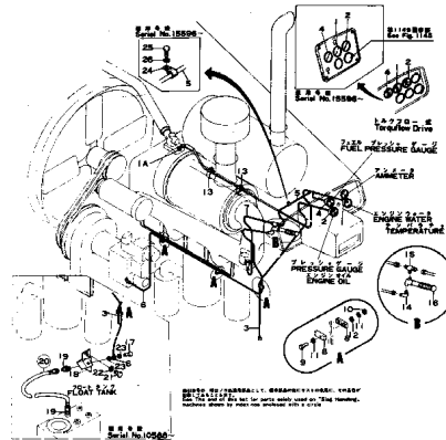
エンジン 関連部品 Fig.1101 ENGINE RELATED PARTS (適用 機種 (Serial No. 10001~ )
