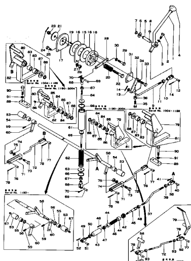
Fig. 104 FUEL CONTROL LEVER (適用機種 Serial No. 1004~5021)
