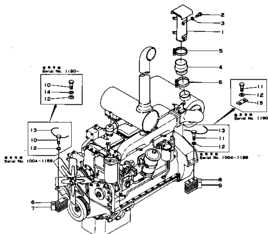
プリクリーナ および エンジン マウント Fig. 101 PRE-CLEANER AND ENGINE MOUNT
