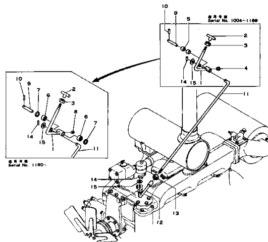
コンプレッション リリース レバー Fig. 103 COMPRESSION RELEASE LEVER
