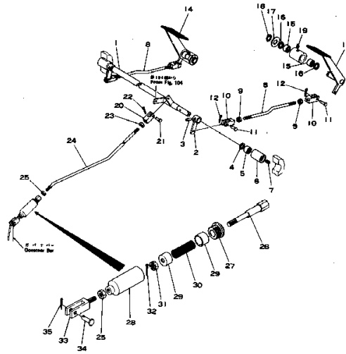
Fig. 105 デセレータペダル (通用号機 DECELERATOR PEDAL (Serial No. 5022~))
