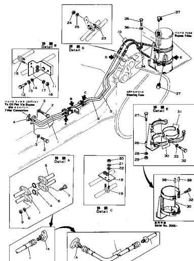
Fig. 102 バイパス フィルタ パイピング BYPASS FILTER PIPING
