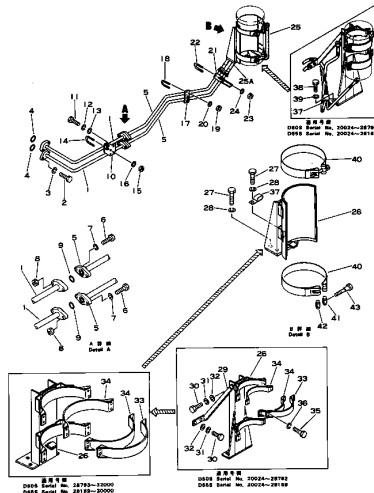
バイパス フィルタ ブラケット および ホース Fig. 1107 BY-PASS FILTER BRAKCT AND HOSE
