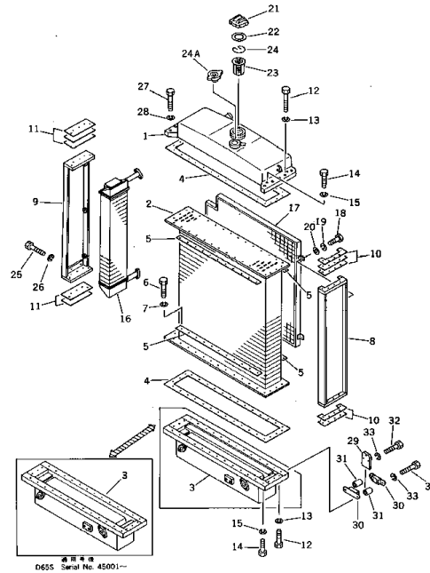
Fig. 131 RADIATOR
