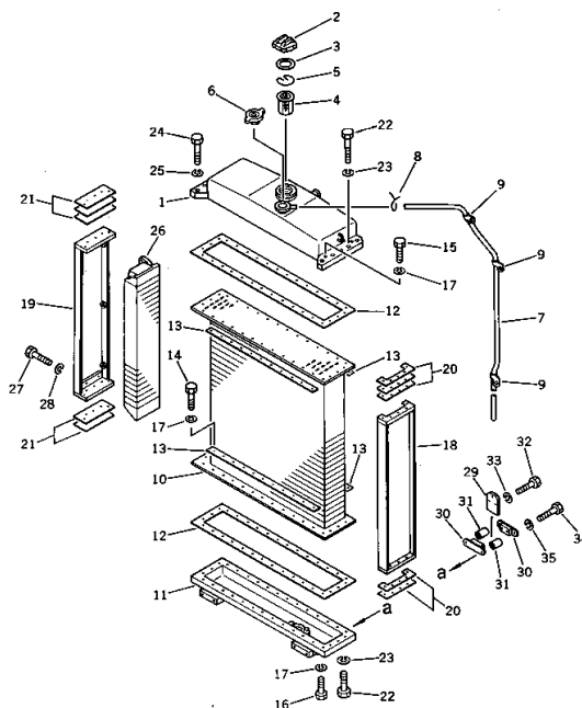
Fig. 131 RADIATOR
