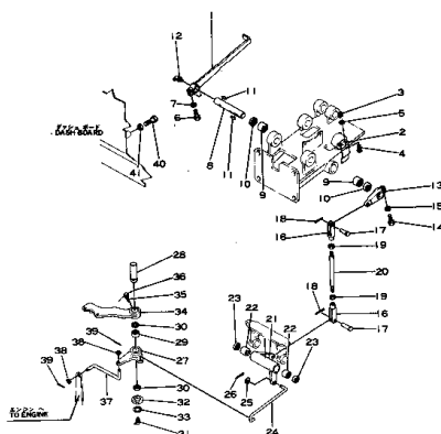
コンプレッション リリース レバー (適用 号機 Fig. 102B COMPRESSION RELEASE LEVER (D60S Serial No. 4656~))
