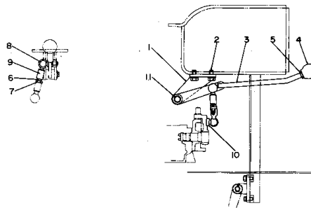
コンプレッション リリース レバー 適用機種 Fig. 102A COMPRESSION RELEASE LEVER (D60S Serial No. 35~1084)
