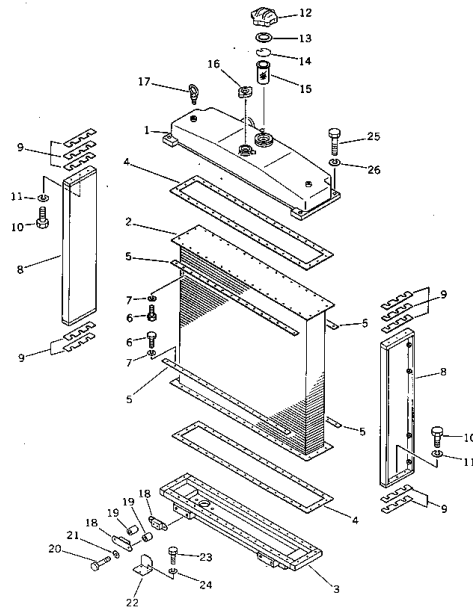
FIG. 132 RADIATOR
