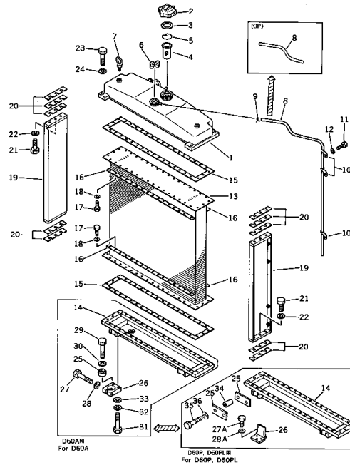
Fig. 131 RADIATOR
