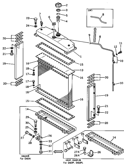
Fig. 131 RADIATOR
