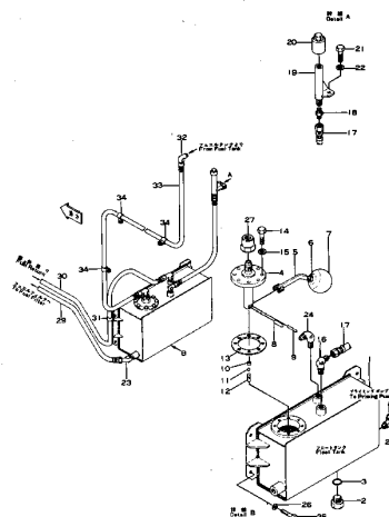
フロートタンク、フューエルホースおよびコネクション Fig. 110 FLOAT TANK, FUEL HOSE AND CONNECTION (適用車種 Serial No. 2005~)
