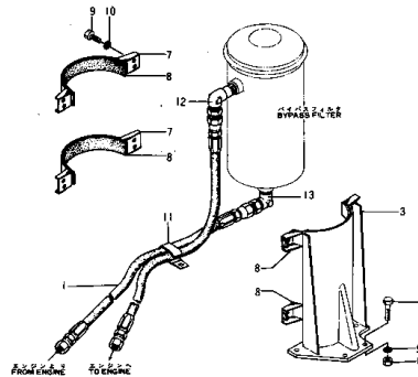
バイパス フィルタ ブラケット および ホース Fig. 109 BYPASS FILTER BRACKET AND HOSE (適用 号 機 (D60P Serial No. 2747-6356)
