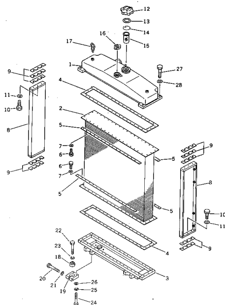
ラジエーター FIG. 131 RADIATOR
