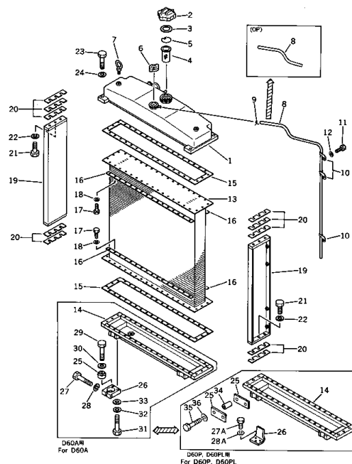
Fig. 131 RADIATOR
