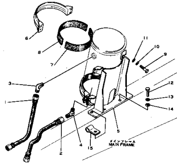
バイパス フィルタ ブラケット 取組 ホース Fig. 107A BYPASS FILTER BRACKET AND HOSE (D60A, P Serial No. 6357~)
