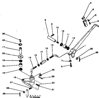
Fig. 101A コンプレッション リリース レバー (D60A,P Serial No. 4542~)
