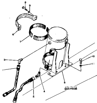
バイパス フィルタ ブラケット および ホース Fig. 107 BYPASS FILTER BRACKET AND HOSE (適用号機 D60A Serial No. 2009-6356)
