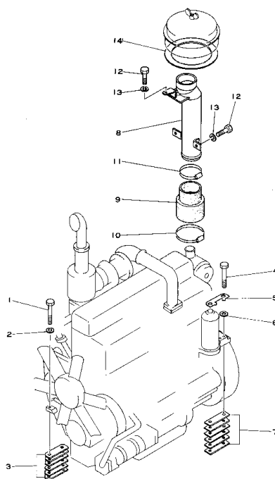
Fig. 101 エンジン 取 付 部 品 ENGINE ATTACHING PARTS
