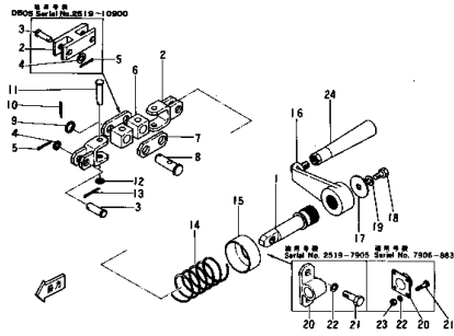
Fig. 102 コンプレッション リリース レバー COMPRESSION RELEASE LEVER (適用 号 機 Serial No. D50S 2519~35000)
