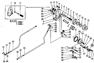
Fig. 103B フュエル コントロール レバー (適用 機種 : D50A, P 10901~35000) (Serial No. D50A, 3771~35000)
