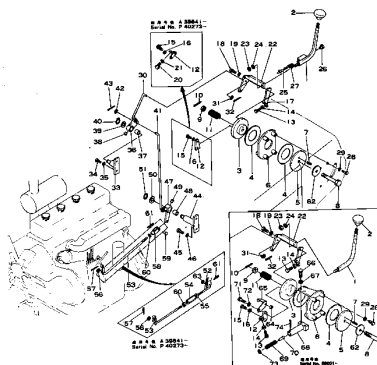
Fig. 1104 フェUEL コントロール レバー (適用 号機 (Serial No. D50A,P,PL 35002~))
