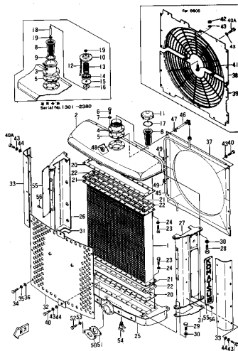
ラジエータ Fig. 121 RADIATOR 通風弁 (Serial No. 4D120 1301--8500)
