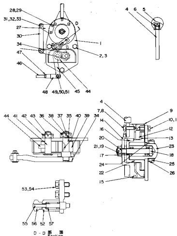
Fig. 103 ファニエル コントロール レバー (適用車種: D50A, P 711~5860) FUEL CONTROL LEVER (Serial No. D50A, P 711~5860) (Serial No. D50S 1201~3770)
