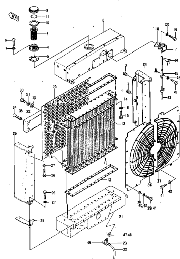
ラジエーター (通角 号機) Fig. 121A RADIATOR (Serial No. 4D120 (10001)~(49999))
