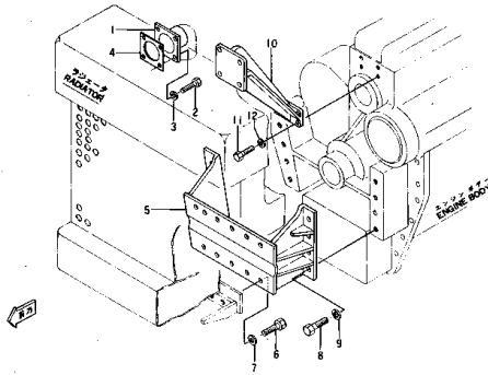
ラジエータ マウンティング (適用 号機 Serial No. 4D120(10001) ~ (49999)) Fig. 122 RADIATOR MOUNTING (Serial No. 4D120(10001) ~ (49999))
