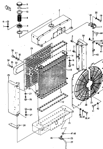
ラジエータ (通称 冷却機) Fig. 121A RADIATOR (Serial No. 4D120 (10001)~(49999))
