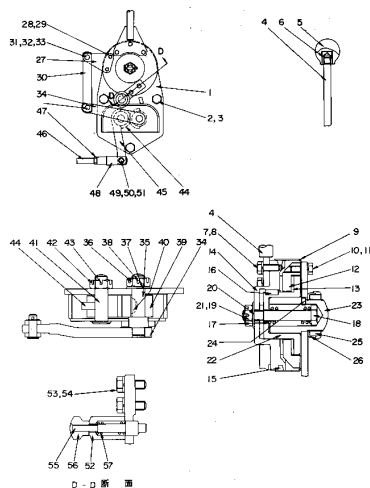
Fig. 103 ファイナルコントロールレバー (適用車種: D50A, P 711~5860) FUEL CONTROL LEVER (Serial No. D50A, P 711~5860) (Serial No. D50S 1201~3770)
