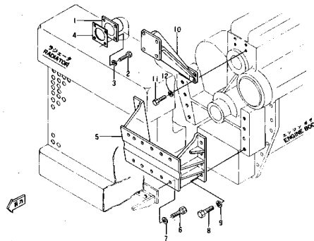
Fig. 122 ラジエータ マウンティング (適用 号機 Serial No. 4D120(10001) ~ (49999))
