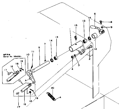
コンプレッション リリース レバー (適用号機 Fig. 1102 COMPRESSION RELEASE LEVER (Serial No. D50A,P,PL 35002-)
