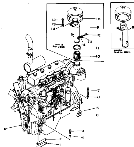
エンジン取付部品 (適用機種) Fig. 1101 ENGINE ATTACHING PARTS (Serial No. 35002~)
