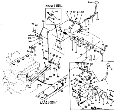
Fig. 1104 フュエル コントロール レバー (適用 機種 Serial No. D50A, P, PL 35002~)
