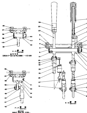
Fig. 105 スターティング ピニオン および クラッチ レバー STARTING PINION AND CLUTCH LEVER (5/6) (適用年表 Serial No. D50A.P 5861-15400)
