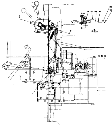
Fig. 104 スターティング ピニオン および クラッチ レバー (適用機種) (Serial No. D50A.P 5861~15400)
