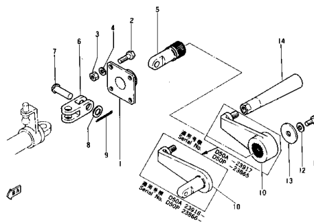
Fig. 101 コンプレッション リリース レバー COMPRESSION RELEASE LEVER (適用号機 Serial No. D50A, P 5861~35000)
