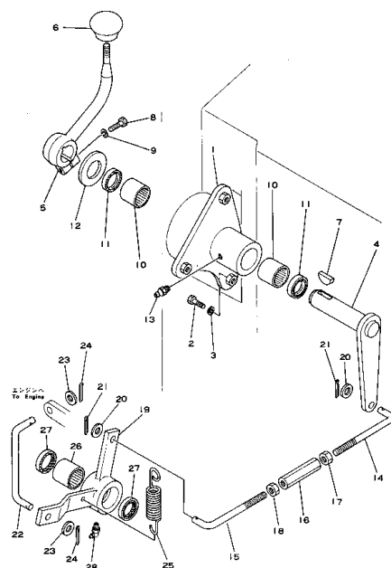
Fig. 111 コンプレッション リリース レバー (適用号機: Serial No. 1501~2200)
