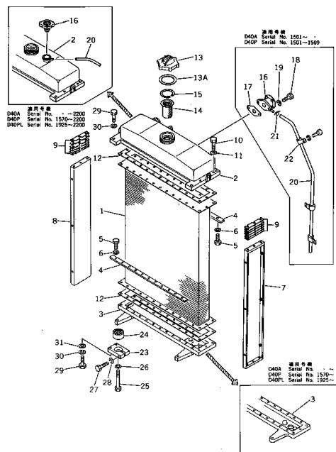
Fig. 131 RADIATOR (適用機種 Serial No. 1501~2200)
