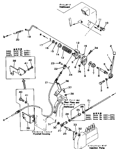
Fig. 121A FUEL CONTROL LEVER (適用号数 Serial No. 2201~)
