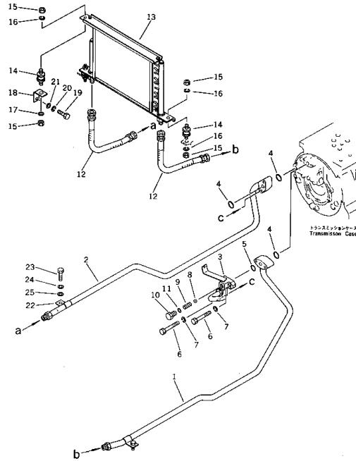
オイルクーラおよびパイピング Fig. 4135 OIL COOLER AND PIPING
