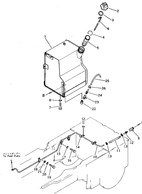
フエルトンク およびパイピング Fig. 4141 FUEL TANK AND PIPING
